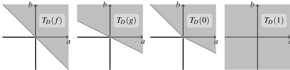
Fig. 12. The Bouligand tangent cones T_D(f) , T_D(g) , T_D(0) and T_D(1) .
